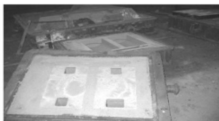
Fot. 3. Odlewy elementu wypełniającego wykonane w masie z udziałem spoiwa Rudal A
