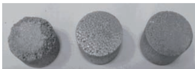
Rys. 35. Wypraski powstałe ze sprasowania mieszaniny proszku Al z gąbką tytanową (95% wag./5% wag.)
