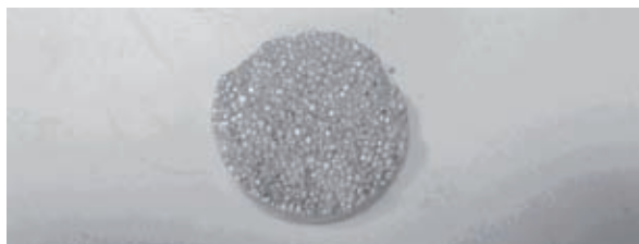
Rys. 36. Wypraski powstałe ze sprasowania mieszaniny proszku Al z gąbką tytanową (85% wag./15% wag.)
