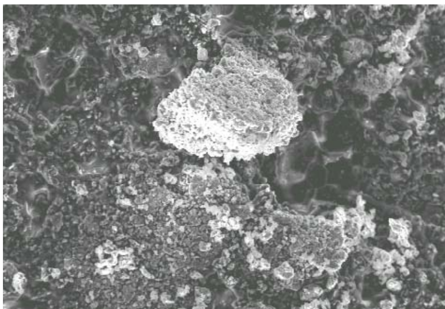
Rys. 12. Próbkę Al-Ti, morfologia badanego materiału, SEM; pow. 800x
