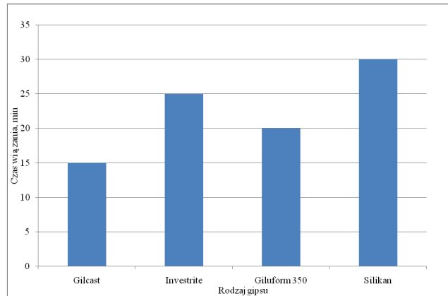
Rys. 5. Czas wiązania badanych gipsów
