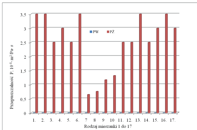
Rys. 6. Badanie przepuszczalności doświadczalnych mas gipsowych 1–17; PW – próbka wilgotna, PZ – próbka wyżarzona
