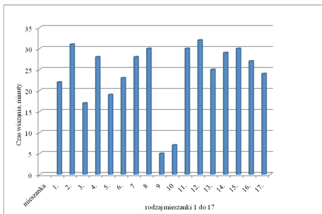
Rys. 9. Badanie czasu wiązania doświadczalnych mas gipsowych 1–17
