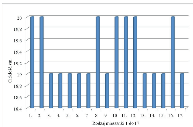
Rys. 8. Badanie ciekłości doświadczalnych mas gipsowych 1–17
