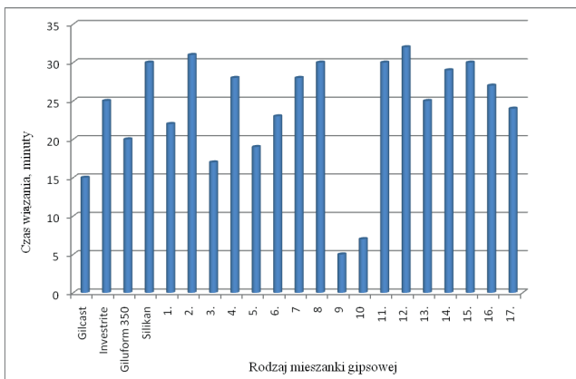
Rys. 14. Porównanie czasu wiązania próbek firmowych oraz opracowanych mieszanek gipsowych 1–17
