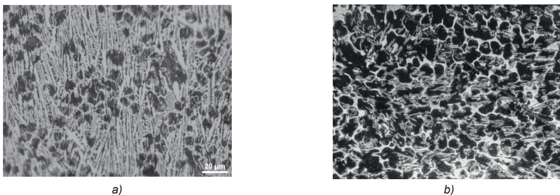
Rys. 2. Mikrostruktura żeliwa białego: a) odlanego grawitacyjnie do formy stalowej, b) odlanego ciśnieniowo, zgląd trawiony nitałem, pow. 500× Fig. 2. White cast iron microstructure: a) gravity die-cast in a steel mould, b) pressure die-cast, specimen etched with nital, 500× magnification
