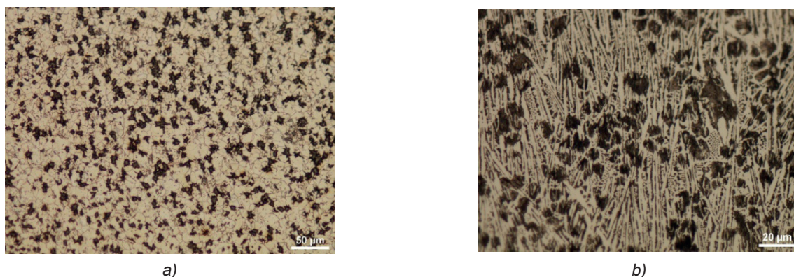
Rys. 3. Mikrostruktura badanego żeliwa po wyżarzaniu grafityzującym: a) pow. 100×, b) pow. 500× Fig. 3. Microstructure of the tested cast iron after graphitising annealing: a) magnif. 100×, b) magnif. 500×
