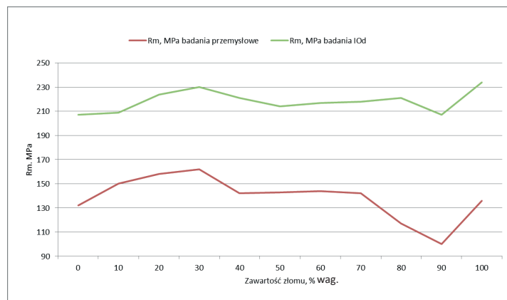
Rys. 15. Porównawcze wyniki badań wytrzymałościowych odlewów ze stopu AZ91 otrzymanych w Instytucie Odlewnictwa (IOd) i w przemyśle
