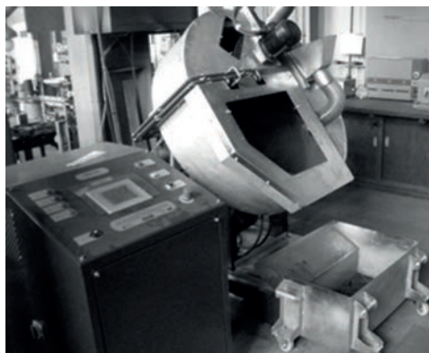
Rys. 2. Granulator misowy, widok ogólny [13] Fig. 2. A general view of the pan-type granulator [13]
