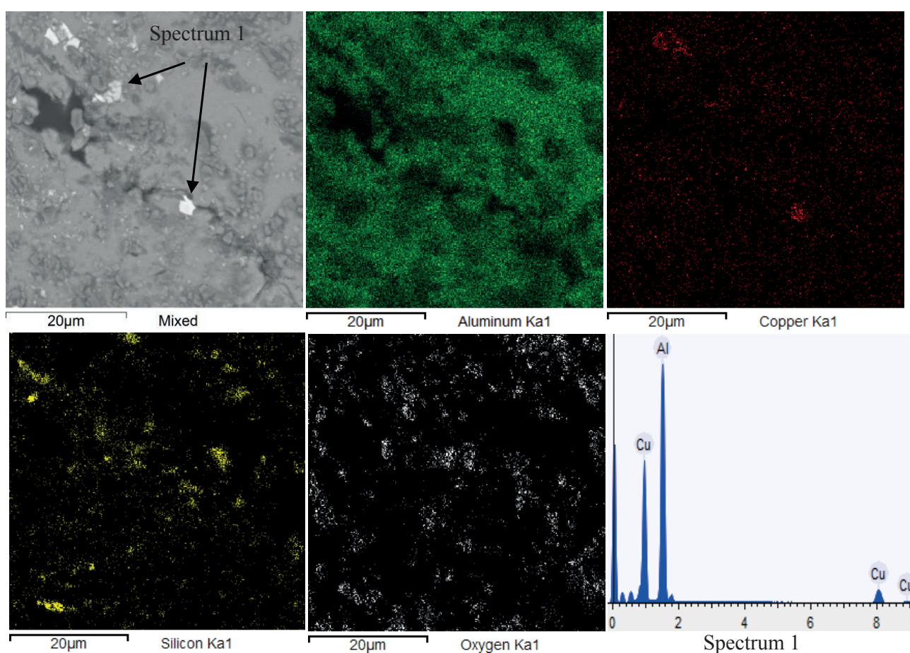
Rys. 7. Rozkład pierwiastków w materiale kompozytowym AW-2024 + 20% obj. cząstek \alpha - \text{Al}_2\text{O}_3 Fig. 7. The distribution of elements in the composite material AW-2024 + 20% vol. of \alpha - \text{Al}_2\text{O}_3 particles
