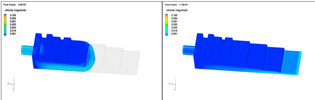
Rys. 14. Wizualizacja wypełnienia matrycy – wariant B: ciśnienie p_1 = 50 kPa, czas wypełnienia 11,5 s, natężenie przepływu 6,85 \text{ cm}^3 \cdot \text{s}^{-1}
