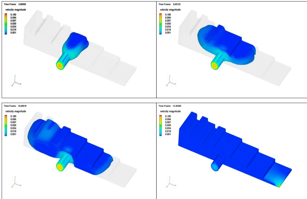
Rys. 13. Wizualizacja wypełnienia matrycy – wariant A: ciśnienie p_1 = 50 \text{ kPa} , czas wypełnienia 12 s, natężenie przepływu 6,6 \text{ cm}^3 \cdot \text{s}^{-1}
