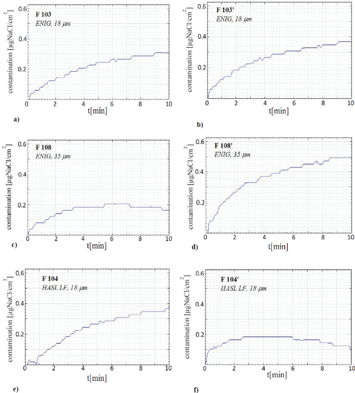
Rys. 5. Zależność zanieczyszczenia jonowego wyrażonego w μg NaCl/cm 2 powierzchni płytek PCB o różnych pokryciach z wlotowanymi komponentami w funkcji czasu: a–b) pokrycie ENIG, grubość warstwy miedzi – 18 μm; c–d) pokrycie ENIG, 35 μm; e–f) pokrycie HASL LF, 18 μm
