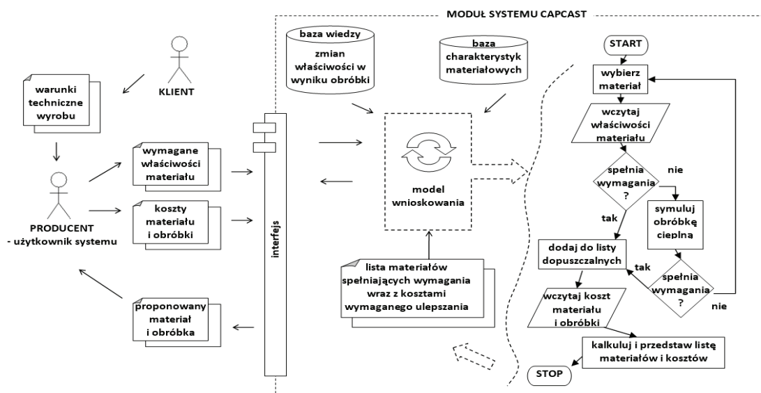
Rys. 1. Schemat modelu wnioskowania dla modułu materiałowego w systemie CAPCAST [1]
