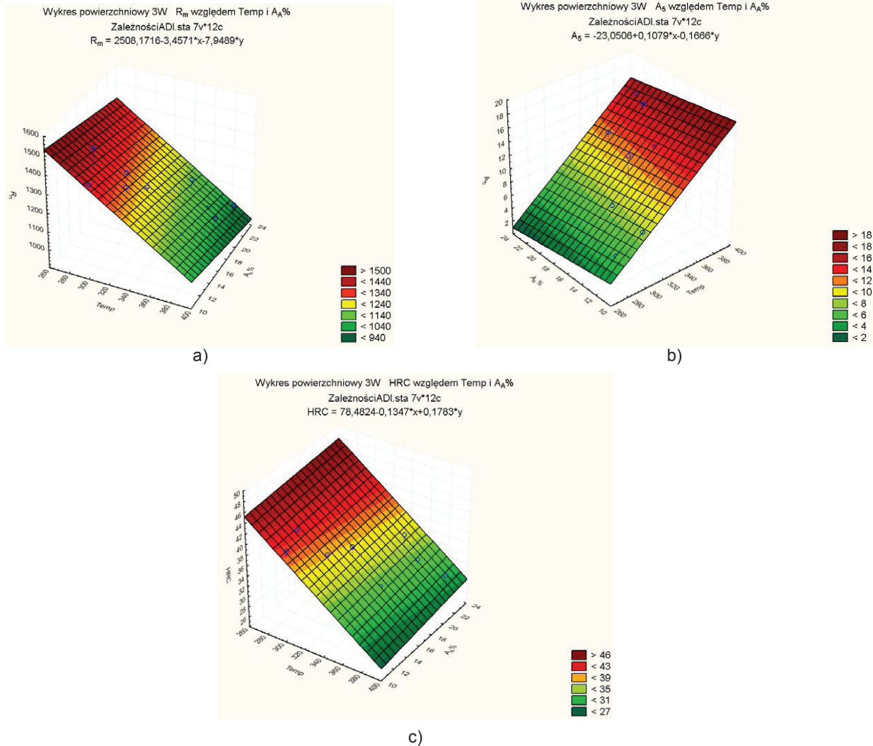
Rys. 7. Wykresy zależności wybranych właściwości żeliwa ADI od temperatury (T) i udziału austenitu w osnowie ( A_A\% ):
