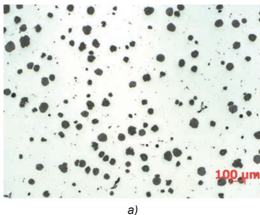
Rys. 2. Mikrostruktura badanego stopu: a) zgład nietrawiony; b) zgład trawiony
