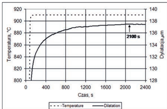
Rys. 4. Określenie czasu austenitizacji stopu
