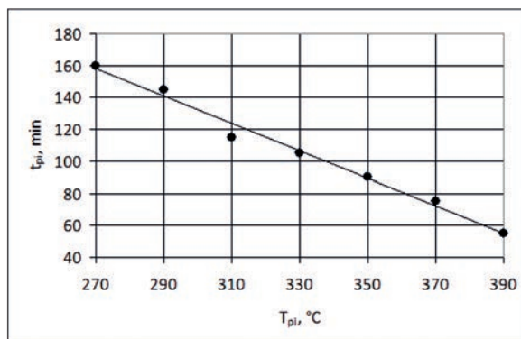
Rys. 9. Określenie parametrów obróbki cieplnej żeliwa sferoidalnego – czasu ausferrytyzacji dla wybranych wartości temperatury przemiany
