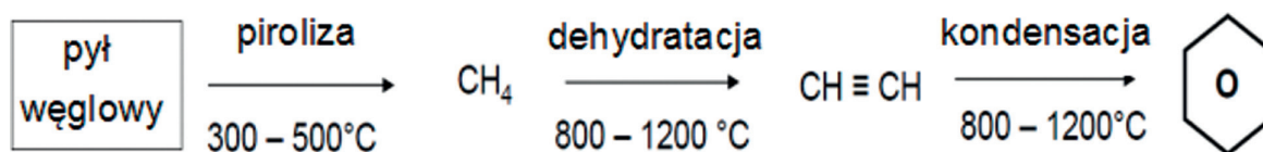
Rys. 1. Schemat tworzenia się benzenu z pyłu węglowego w wyniku rekombinacji (800–1200°C) [11]
