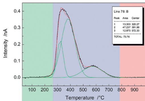
Rys. 4. Zakres wydzielalności benzenu z mieszanki bentonit + NWB [19]
