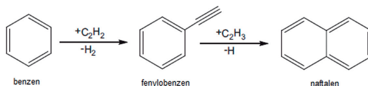
Rys. 7. Mechanizm tworzenia się naftalenu z benzenu [25]
