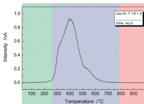
Rys. 5. Zakres wydzielalności toluenu, etylobenzenu i ksilenów z mieszanki bentonit + NWB [19] Fig. 5. Range of toluene, ethylbenzene and xylene emittability from the bentonite + LCF mixture [19]
