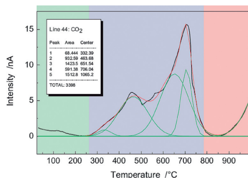
Rys. 2. Zakres wydzielalności CO 2 z mieszanki bentonit + NWB [19]
