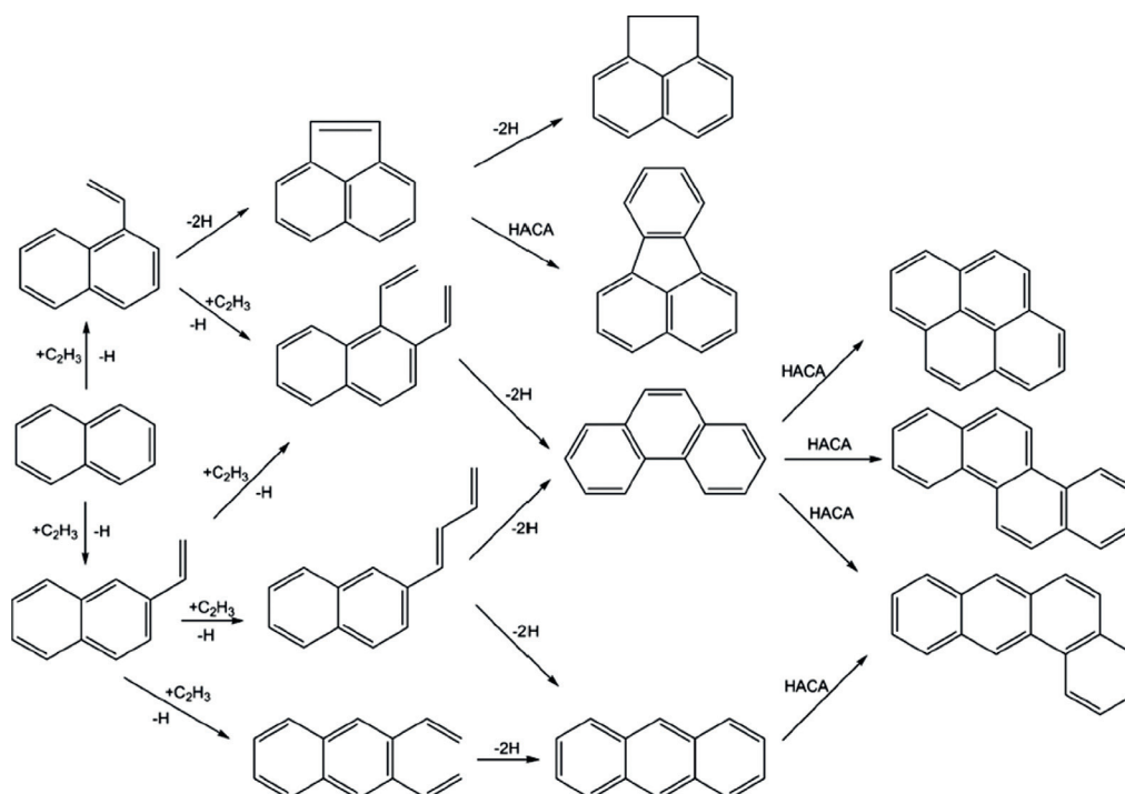
Rys. 8. Mechanizm tworzenia się trzy- i czteropierścieniowych węglowodorów aromatycznych [25]
