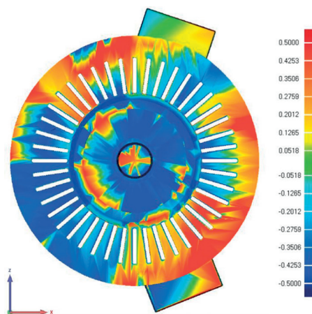
Rys. 13. Wyniki kontroli wymiarowej rdzenia przedstawione na widoku z dołu – wartości w mm Fig. 13. The results of the core dimensional control presented on the bottom view – the values in mm
