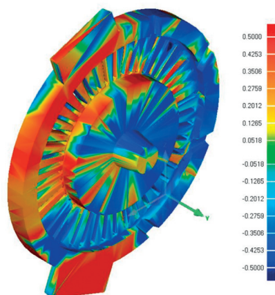
Rys. 12. Wyniki kontroli wymiarowej rdzenia przedstawione na widoku izometrycznym – wartości w mm Fig. 12. The results of the core dimensional control presented on isometric view – values in mm
