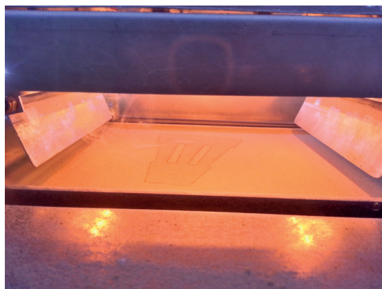
Rys. 4. Widok urządzenia LS ONE podczas wykonywania elementu rdzenia
