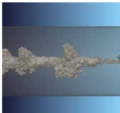
Rys. 14. Wizualizacja 3D wad skurczowych w odlewach testowych stopu IN740 Fig. 14. 3D visualisation of shrinkage defects in IN740 alloy test castings
