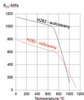
Rys. 7. Charakterystyka termiczna wytrzymałości na rozciąganie stopu H282
