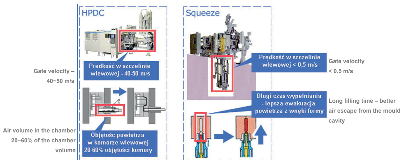
Rys. 6. Porównanie prędkości wypełniania wnętrza formy w technologii HPDC i HSC [17]
