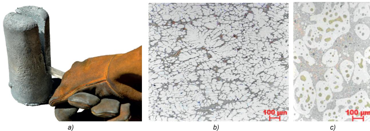
Rys. 14. Wlewek ze stopu AlSi7Mg otrzymany metodą Rheocast (a), mikrostruktura odlewu kokilowego ze stopu AlSi7Mg (b) oraz po sprasowaniu w stanie ciekłym, sprzyjającym globularyzacji faz i wydzielań (c)
