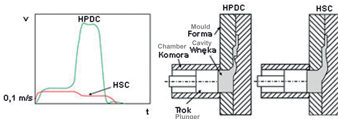
Rys. 7. Różnica w prędkości wypełniania wnętrza formy (a) oraz różnica w wielkości szczeliny wlewowej w obu technologiach (b) [18]
