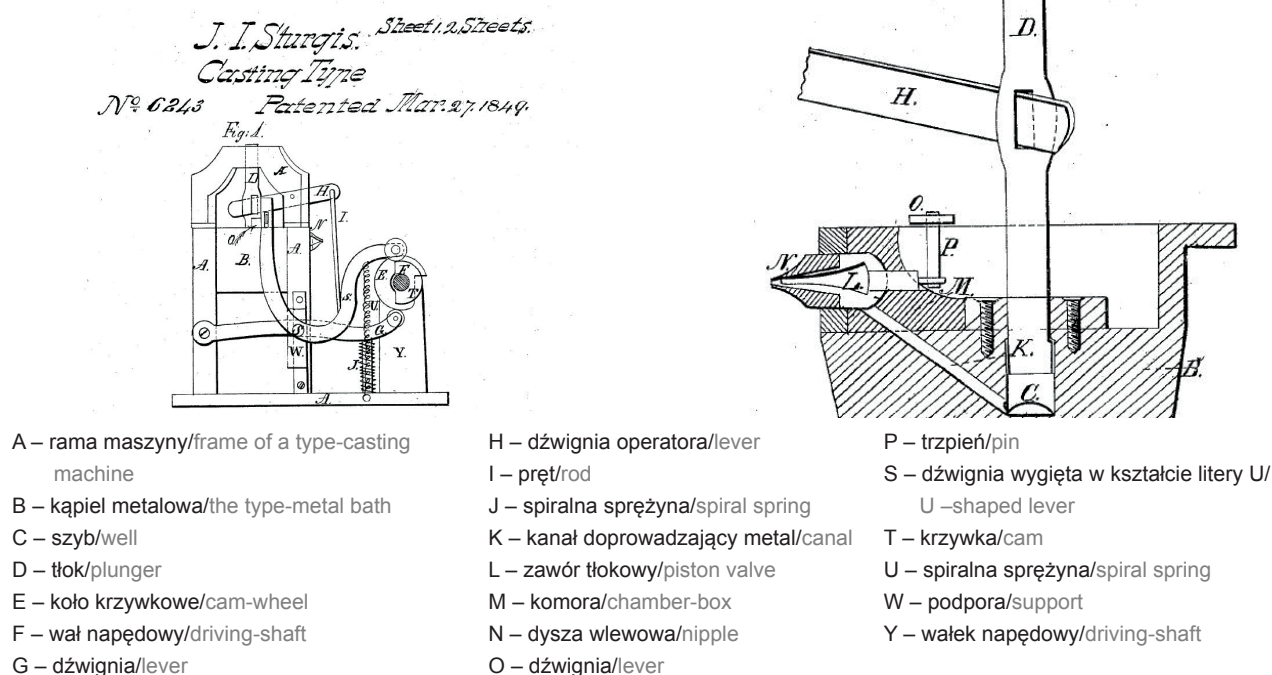
Rys. 2. Schemat maszyny do odlewania czcionek drukarskich (według opisu patentowego Johna I. Sturgisa [5]) Fig. 2. A schematic diagram of a type-casting machine (According to the patent description of John I. Sturgis [5])
