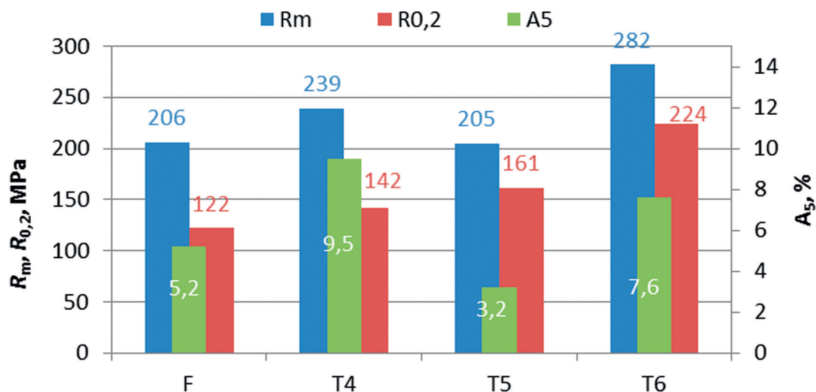
Rys. 15. Właściwości mechaniczne odlewów ze stopu AlSi7Mg prasowanych w stanie ciekłym po obróbce cieplnej (badania własne – zrealizowane w ramach projektu ZAMAT). Właściwości wytrzymałościowe wyznaczano na próbkach wycinanych z odlewu
