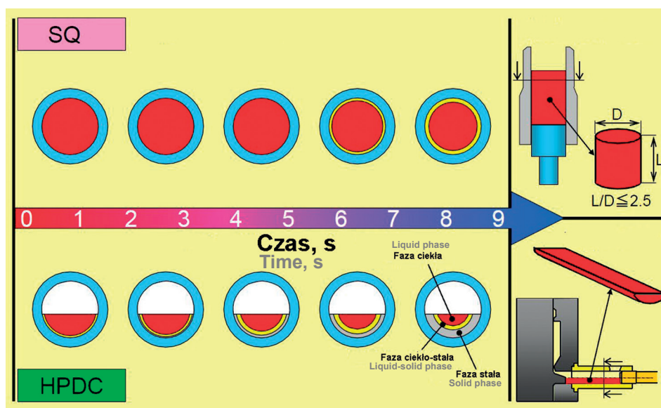
Rys. 3. Porównanie stopnia wypełnienia wnętrza formy w przypadku prasowania w stanie ciekłym (na górze) oraz w przypadku odlewania pod wysokim ciśnieniem (u dołu) [11]
