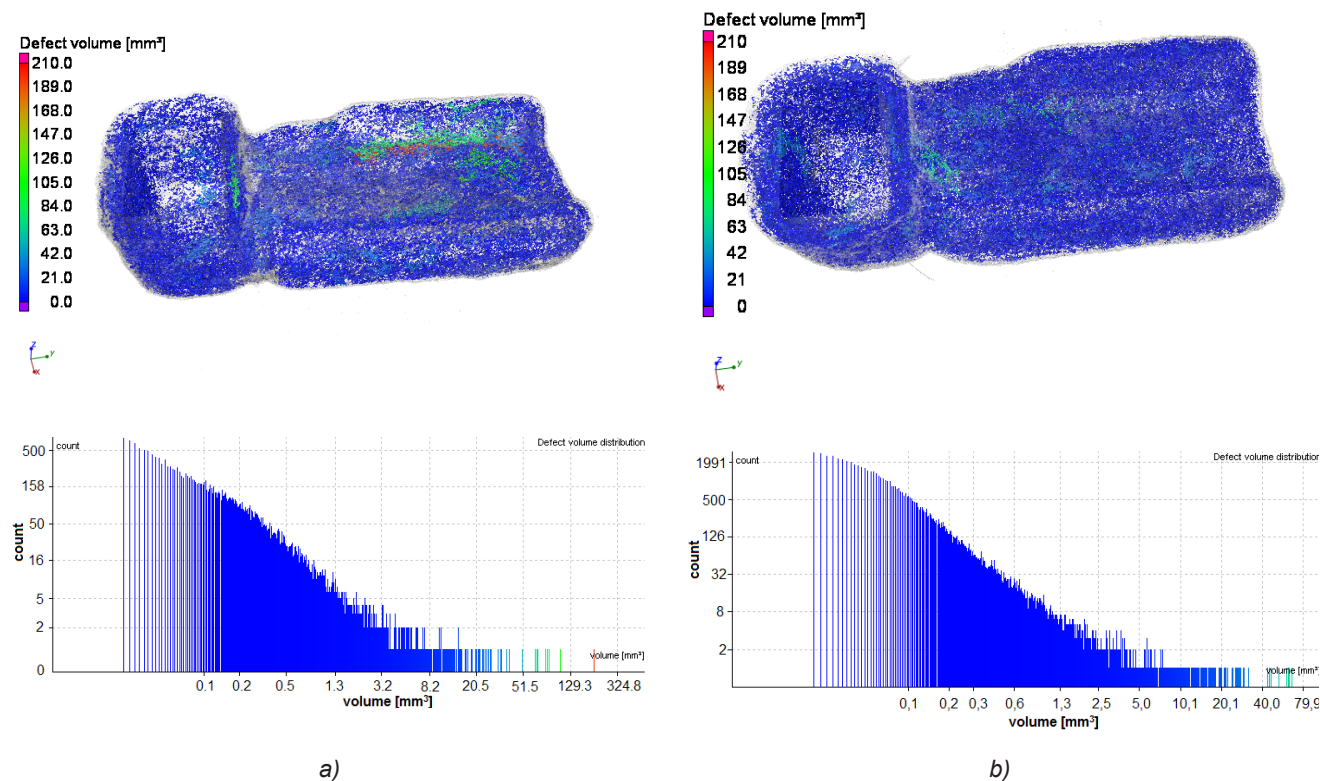
Rys. 5. Przykładowa przestrzenna wizualizacja porowatości w formie typu A (a) i B (b)
