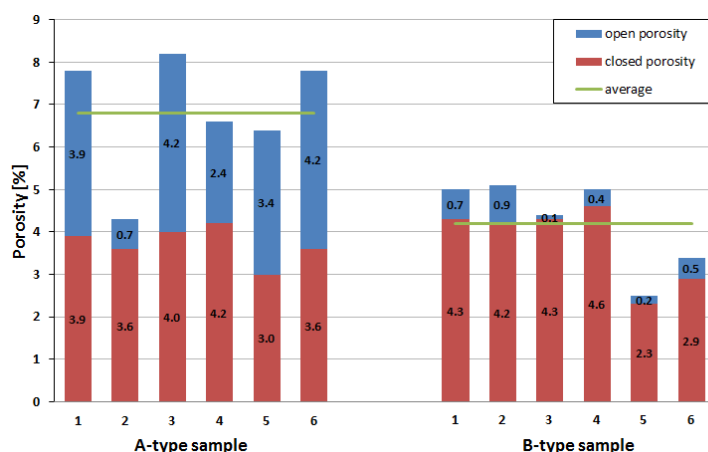
Rys. 4. Procentowy udział porowatości w poszczególnych próbkach typu A i B
